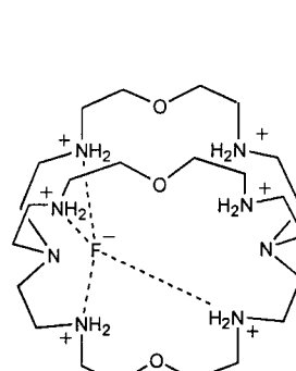
bis-tren(F) A
